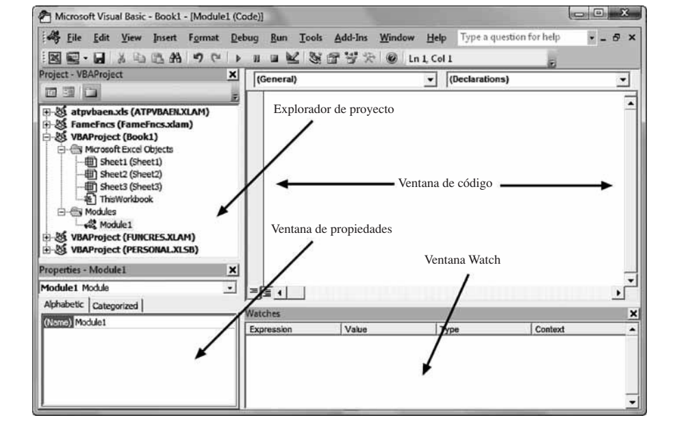
FIGURA 14-2 EL EDITOR VISUAL BASIC
