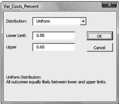
FIGURA 12-10 CUADRO DE DIÁLOGO DE DISTRIBUCIÓN PARA COSTOS VARIABLES
