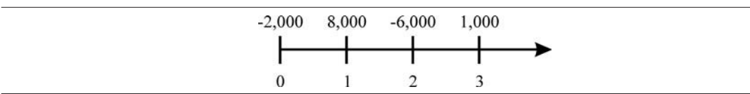
FIGURA 11-3 FLUJOS DE EFECTIVO PARA IRR MÚLTIPLES
