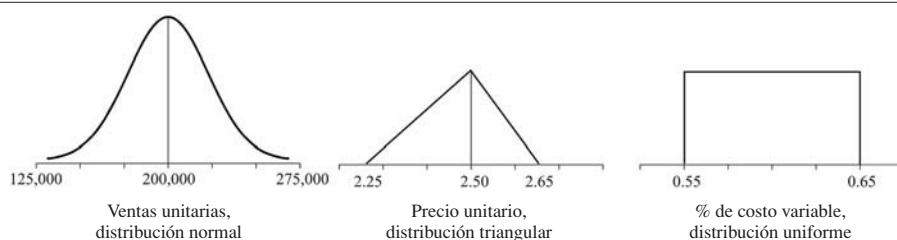
FIGURA 12-6 GRÁFICAS DE DISTRIBUCIONES DE PROBABILIDAD
