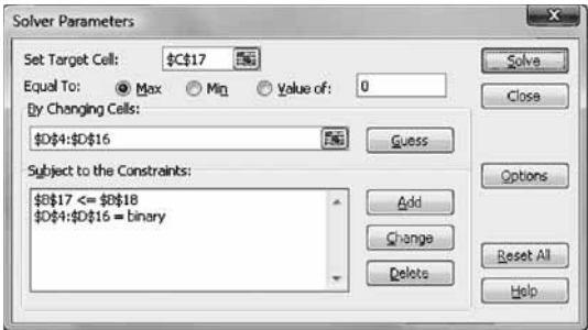
FIGURA 11-9 CUADRO DE DIÁLOGO DE SOLVER
