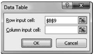
FIGURA 12-3 CUADRO DE DIÁLOGO DE TABLA DE DATOS
