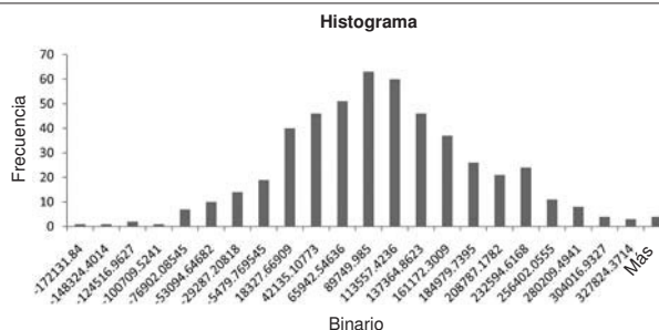
HISTOGRAMA DE LOS NPV DE LA SIMULACIÓN
