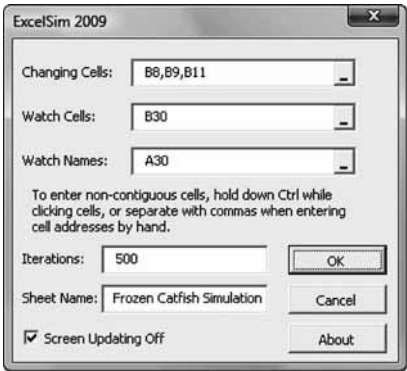
FIGURA 12-7 CUADRO DE DIÁLOGO PRINCIPAL EXCELSIM
