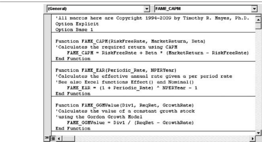
FIGURA 14-4 LA VENTANA DE CÓDIGO
