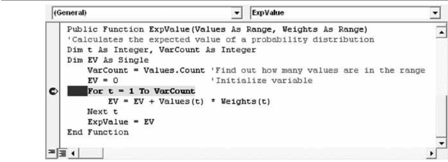
FIGURA 14-8 VENTANA DE CÓDIGO CON UN PUNTO DE RUPTURA
