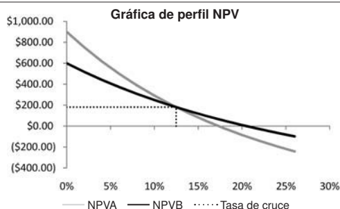
FIGURA 11-6 GRÁFICA DE PERFIL NPV PARA DOS PROYECTOS
