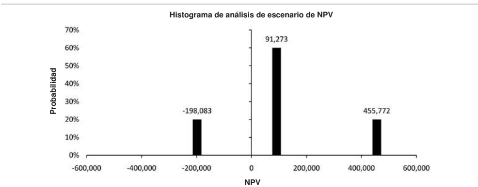
FIGURA 12-5 DISTRIBUCIÓN DE PROBABILIDAD DE NPV
