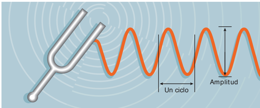
Figura 3-15 Ondas sonoras.
