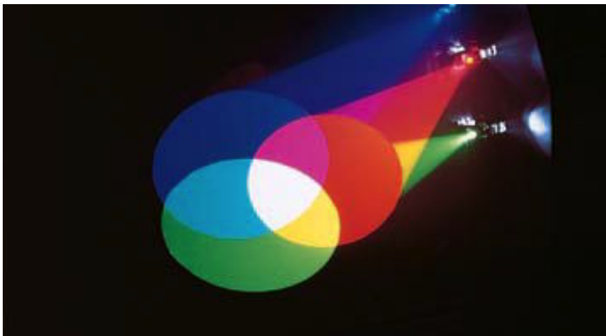
Figura 3-11 Mezcla aditiva de colores.
