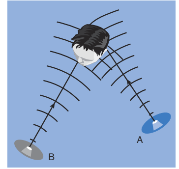
Figura 3-32 Señales empleadas para localizar el sonido.
